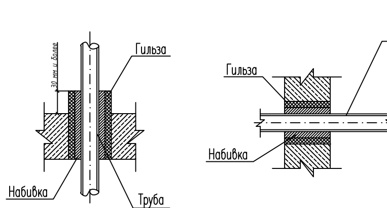
Прокладка трубопроводов системы отопления через стены, перегородки и перекрытия
