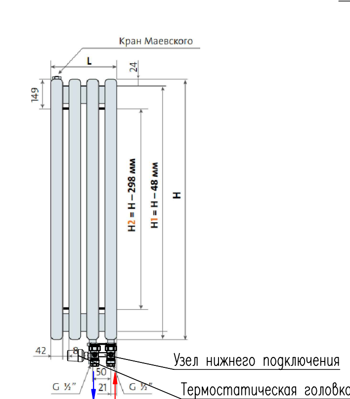
Узел обвязки высокого вертикального трубчатого радиатора
